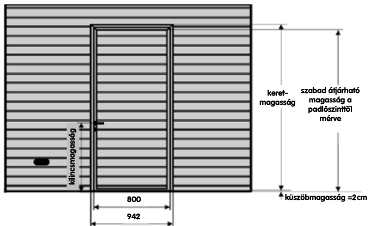
Alacsony küszöbös kisajtó, 800mm alap szélességben
