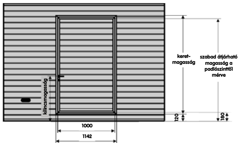
Alacsony küszöbös kisajtó, 1000mm szélesített változatban
